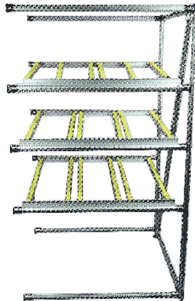
Följesektion
